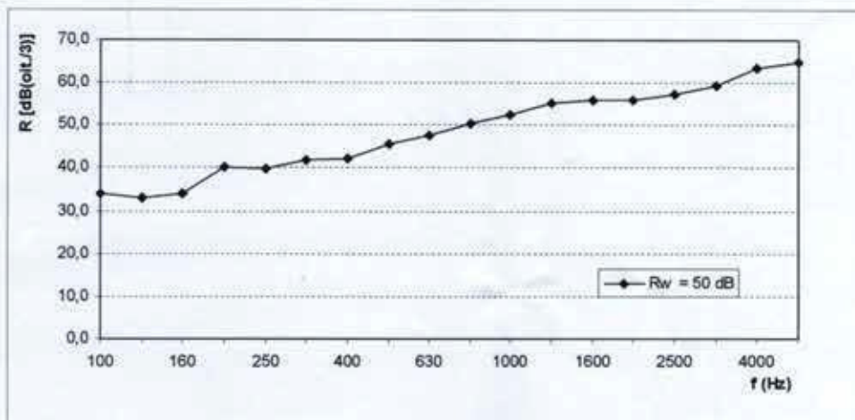
Curva característica de isolamento a sons aéreos
